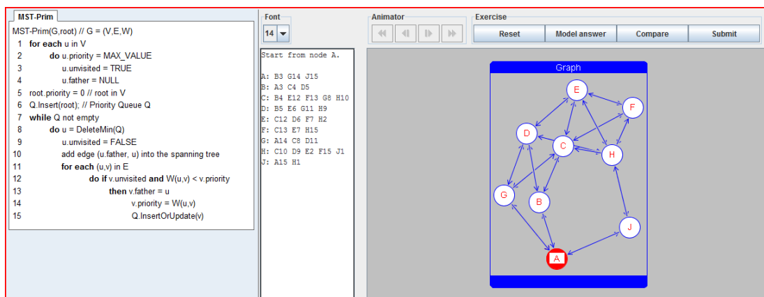
4. ábra. Példa gráfalgoritmusra
