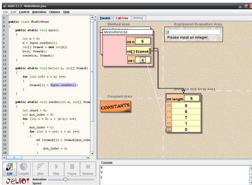
1. ábra. Jeliot
